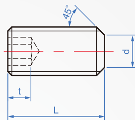
B 平尾形
