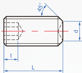
A 杯尾形
