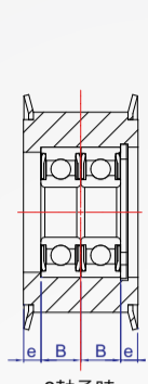
2軸承時
