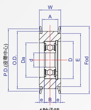
1軸承時
