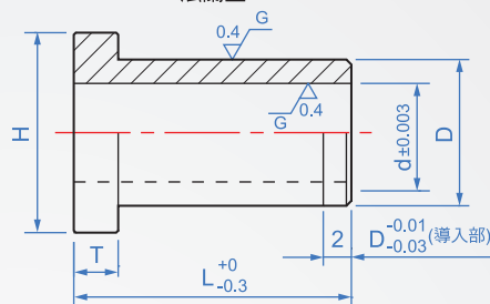
法蘭型
