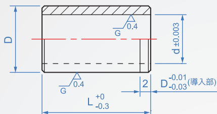
直柱型
