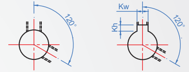
■ Shaft hole P, N size table
