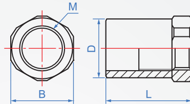
Flange : M14~36
