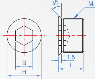
皿座付型
